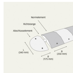
Richtstange, für Fahrbahnschwelle Ref. TOPSTOP-ROHR
