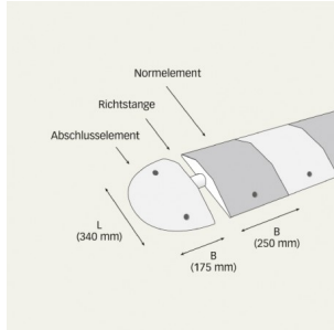
Richtstange, für Fahrbahnschwelle Ref. TOPSTOP-ROHR
